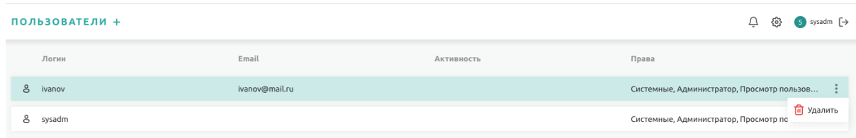
Рис. 3.14. Удаление пользователя
