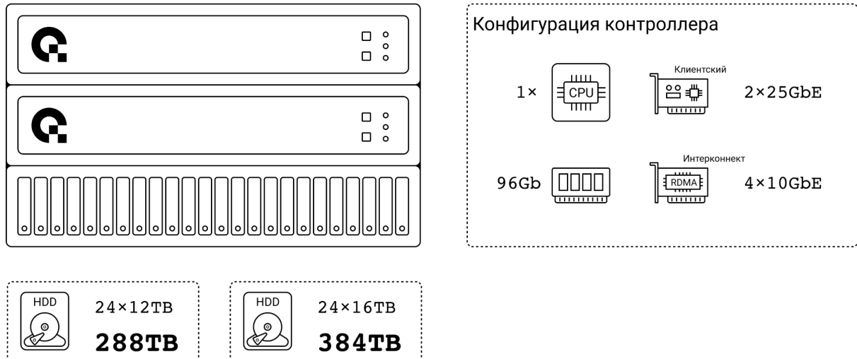
Рис. 5.2. ALL HDD x 24
